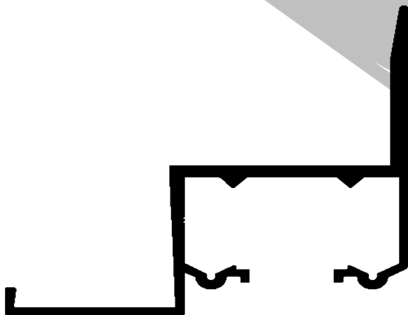
26008 Riel Superior Exterior
